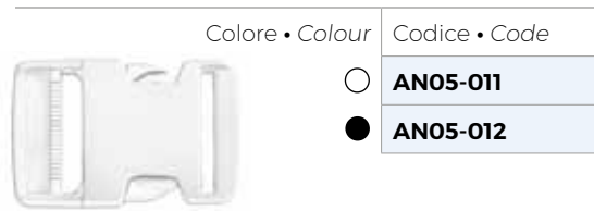
Fibbia a scatto rapido in resina acetilica per nastro da 25mm Snap buckle acetal resin for 25mm tape
