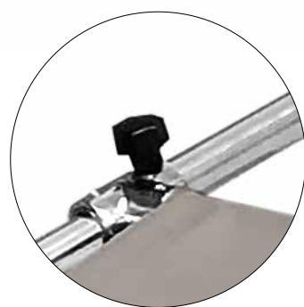
2 Telaio Estraibile Frame Pull-out Bimini Top
